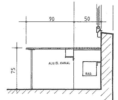
SCHNITT C-C
