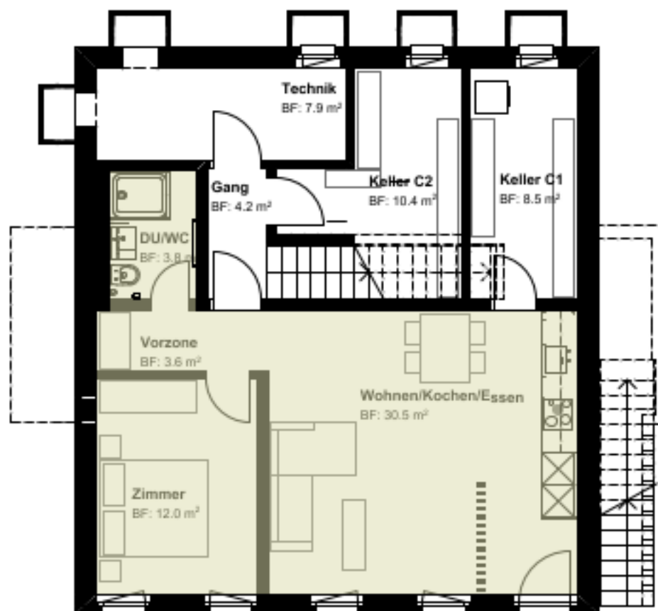
Wohnung C1 2 1/2 Zi.-Whng. BWF: 51.5 m² NWF: 50.2 m²
