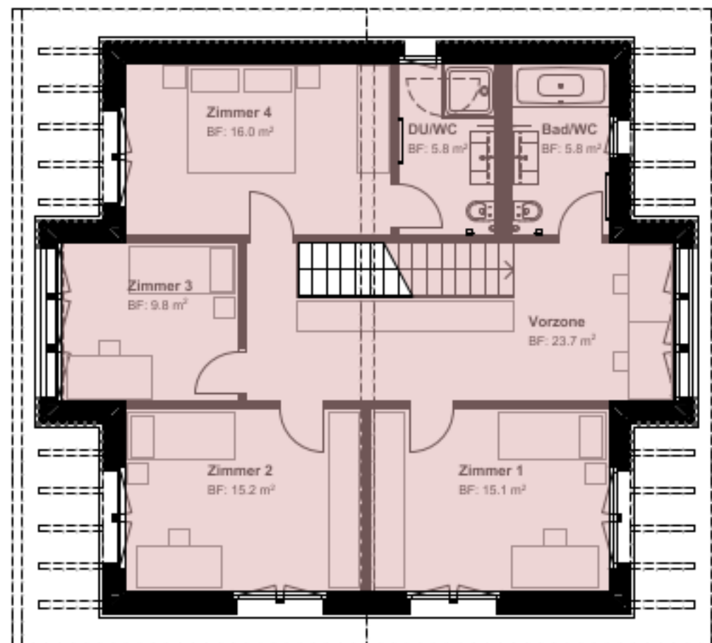
Wohnung C2 Dachgeschoss
