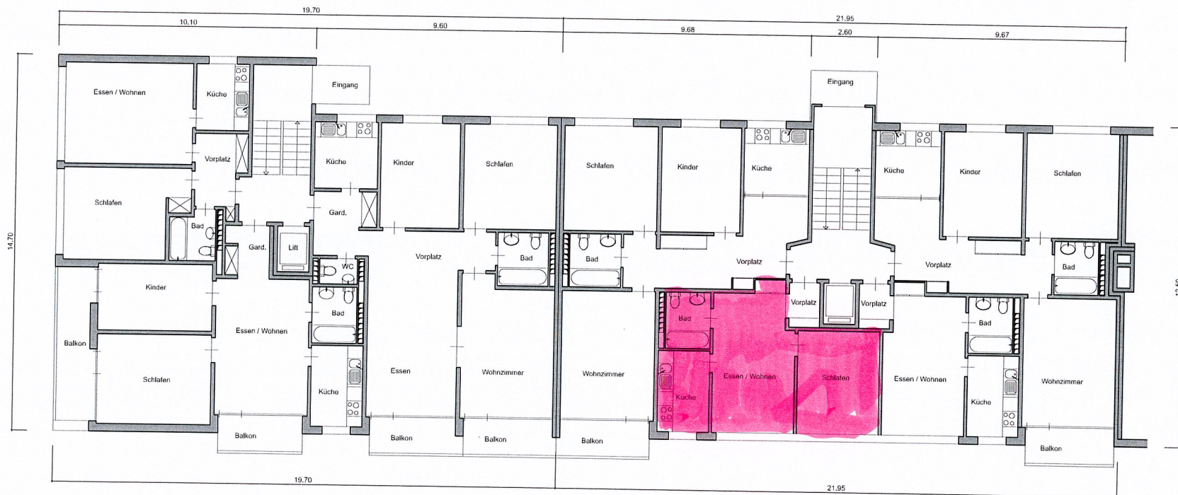
Eckhaus A Grundriss EG
