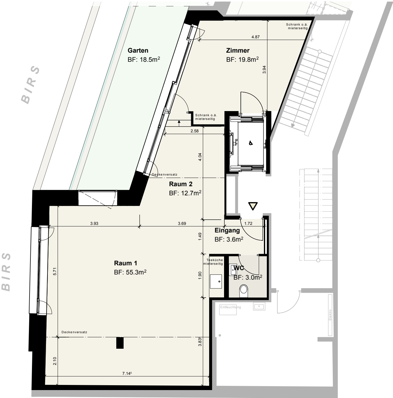
Grundriss Sockelgeschoss, 1:100
