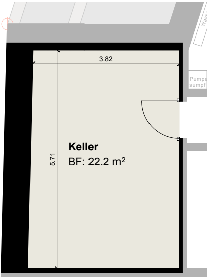
Grundriss Untergeschoss, 1:100
