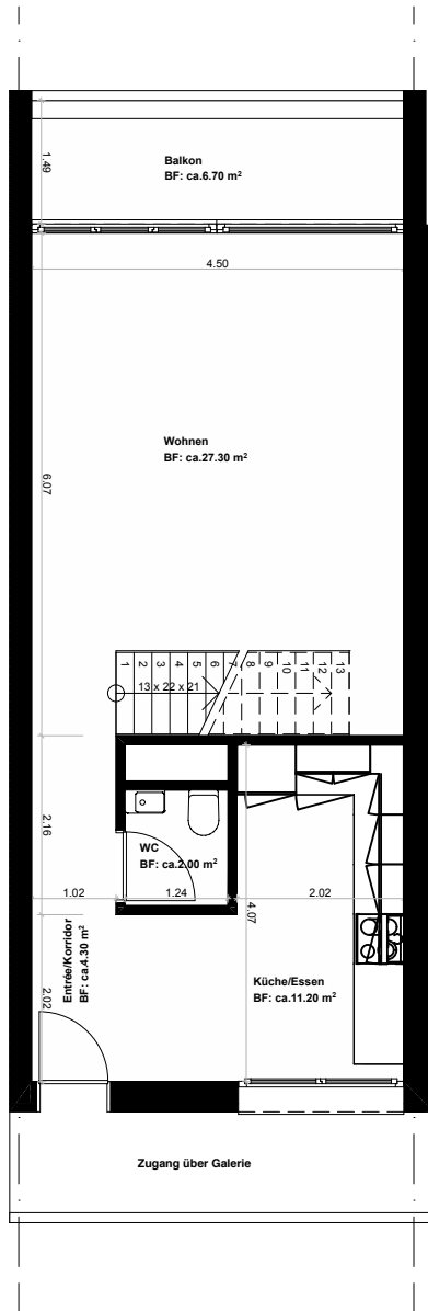
0. 11. Obergeschoss 1:100
