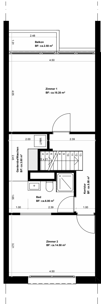
1. 12. Obergeschoss 1:100
