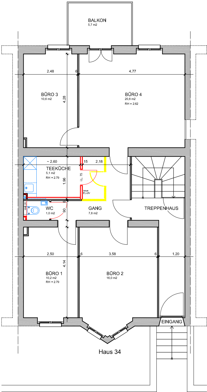
ERDGESCHOSS
