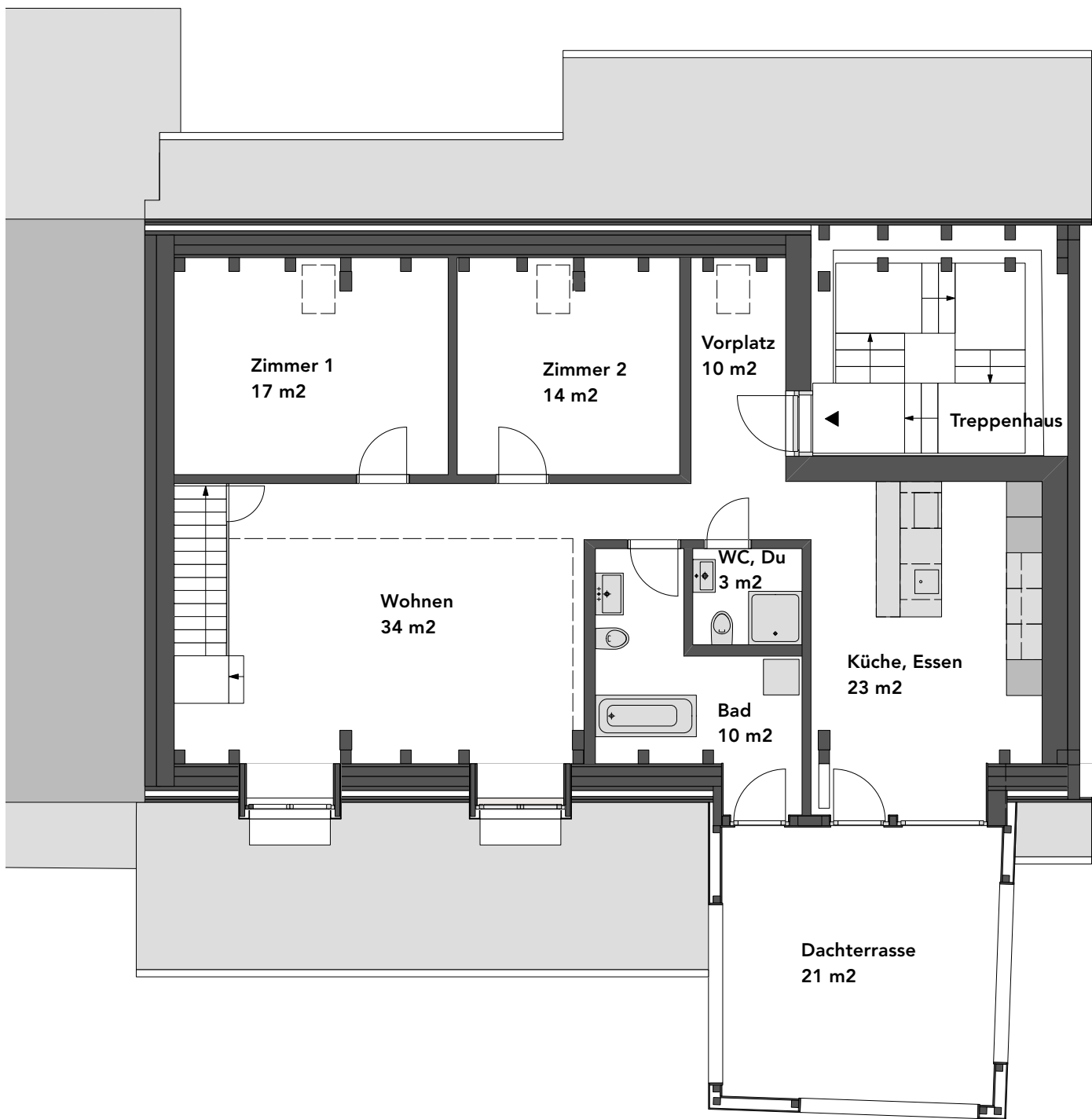
Grundriss Wohnung 3, Dachgeschoss, Säckingerhof 2, Mumpf
