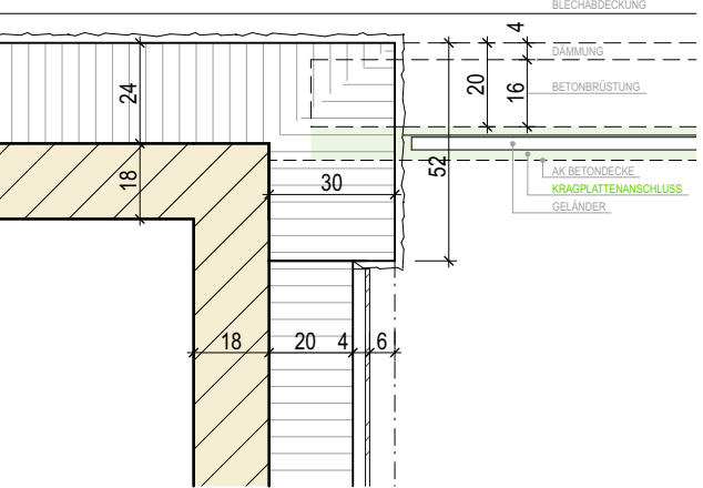
DETAIL 1 : 20
