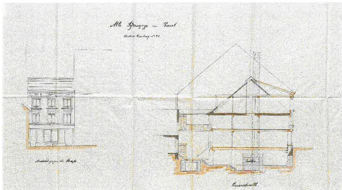
Abb. 2 – Umbau der «Alten Synagoge» zum Wohnhaus mit Bäckerei, Fassade und Querschnitt (Baubegehren 1877, StABS, Bauplanausgabe Unterer Heuberg 21, 1877-482)
