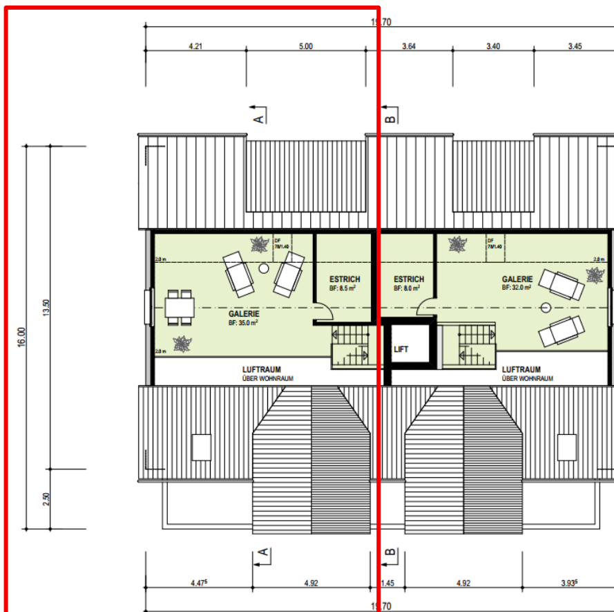
GALERIEGESCHOSS
