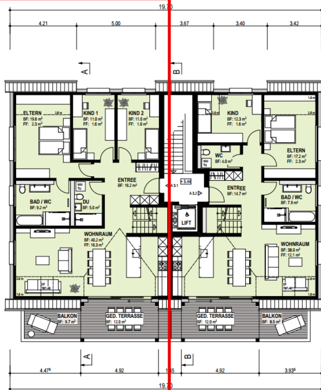
DACHGESCHOSS
