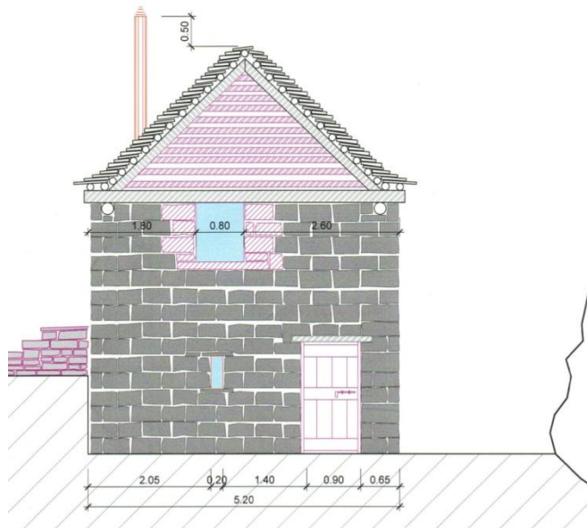
Facciata Sud-Est 1:50
