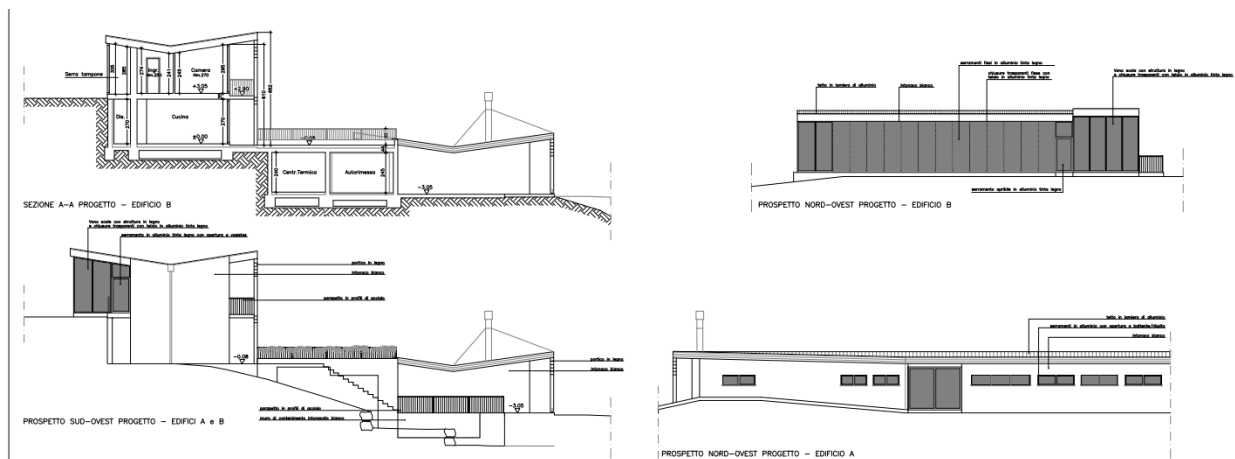
Plan Villa in Konstruktion / planimetria villa in costruzione
