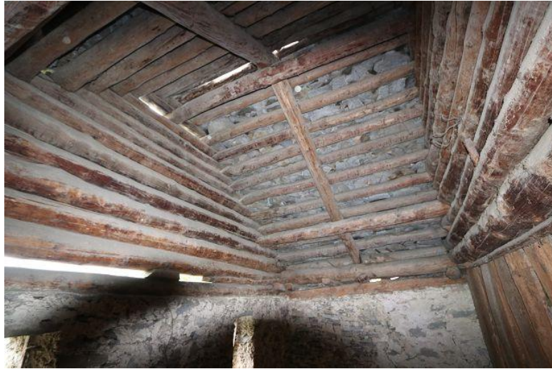
Dachkonstruktion / sotto tetto
