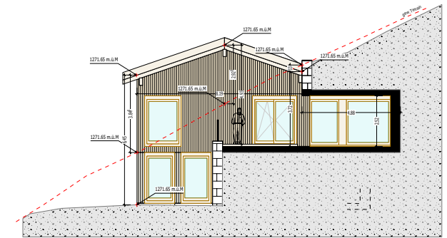
Ostfassade
