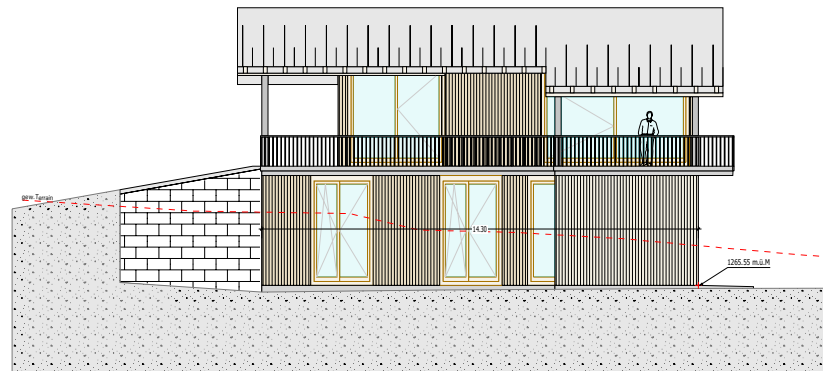
Südfassade
