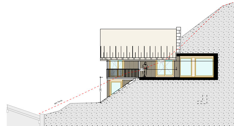
Ostfassade
