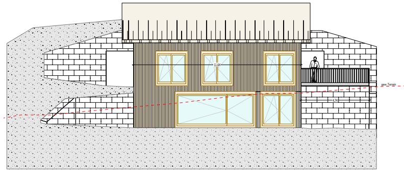
Südfassade
