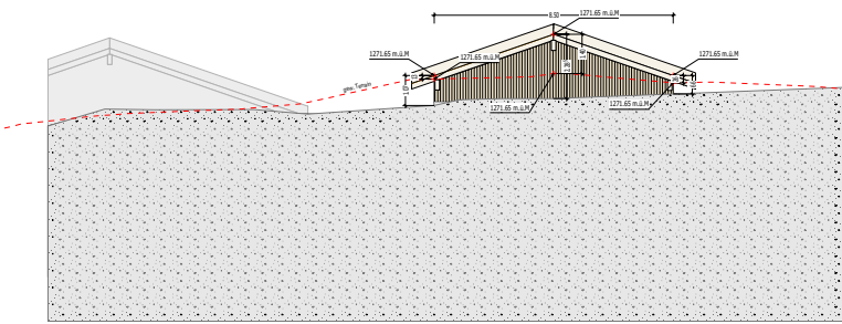
Nordfassade
