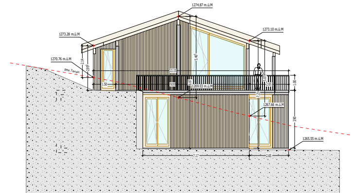
Westfassade
