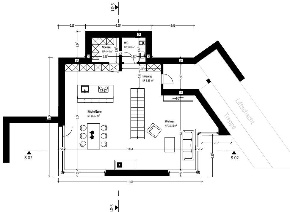
Grundriss Untergeschoss
