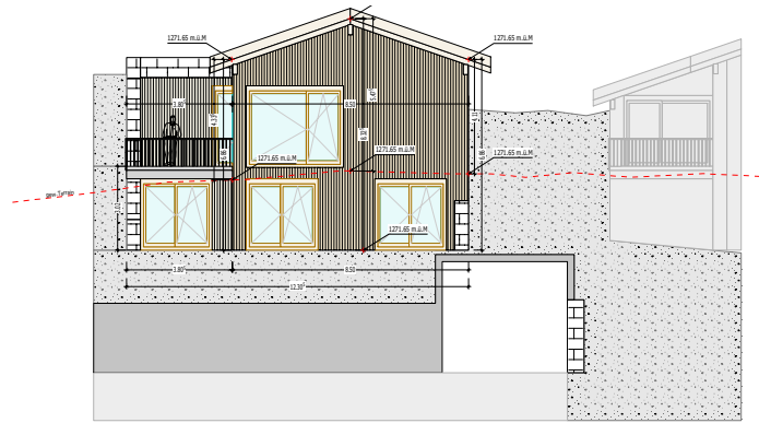
Südfassade
