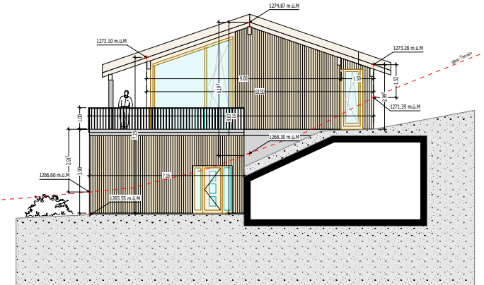
Ostfassade
