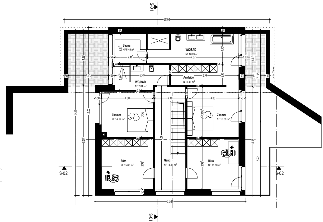
Grundriss Obergeschoss
