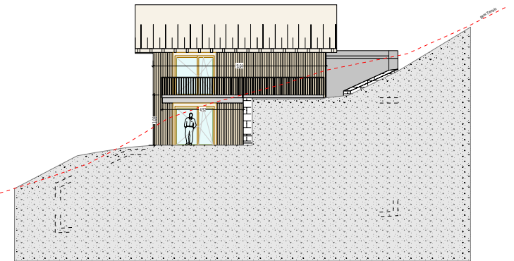
Ostfassade
