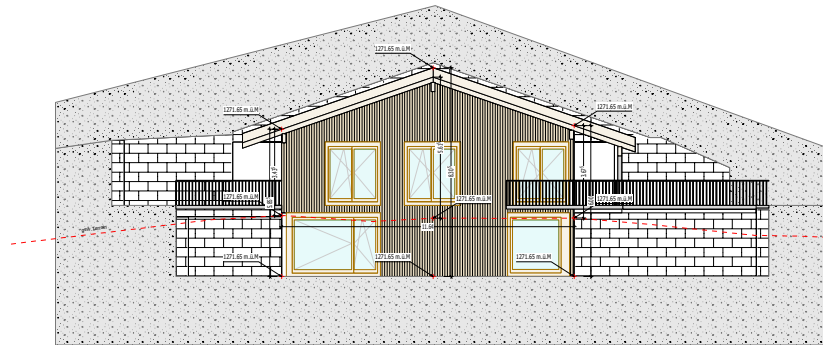
Südfassade
