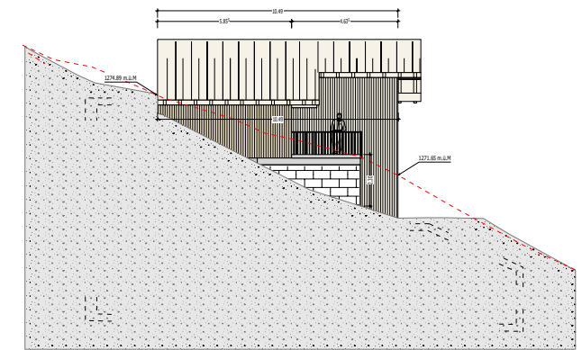
Westfassade
