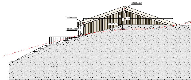
Nordfassade
