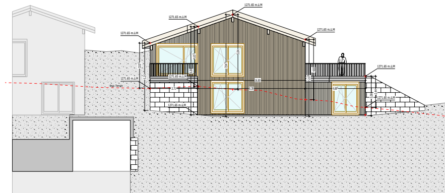
Südfassade
