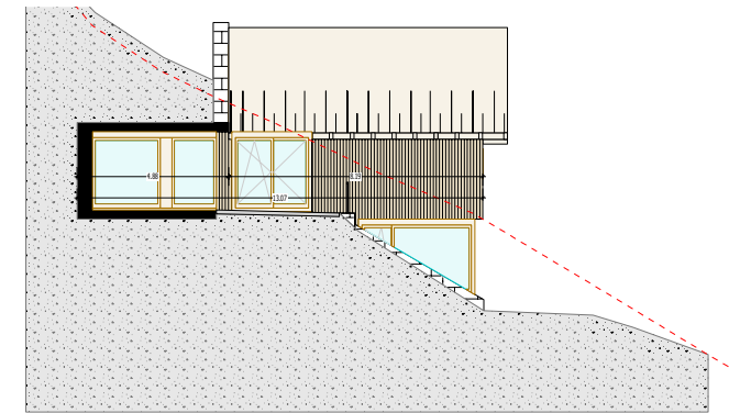
Westfassade
