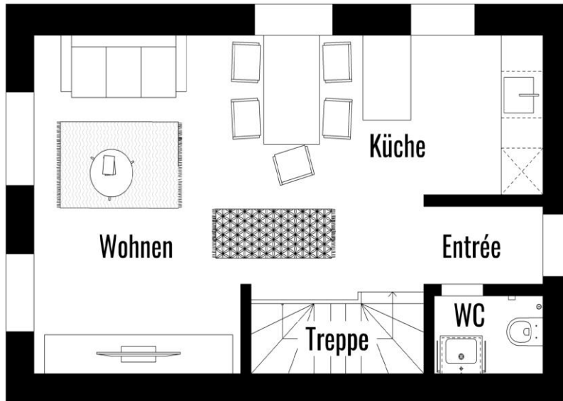
Grundriss Obergeschoss
