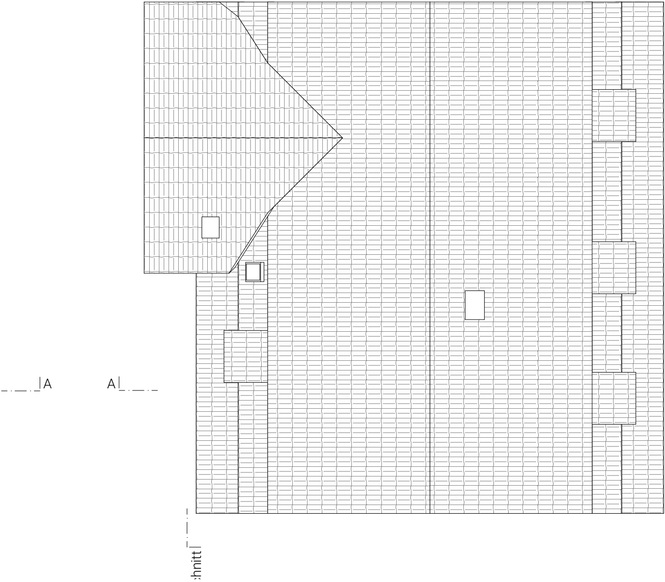
Grundriss Dachaufsicht
