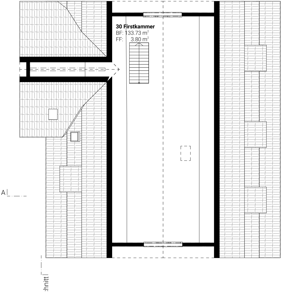
Grundriss Dachgeschoss
