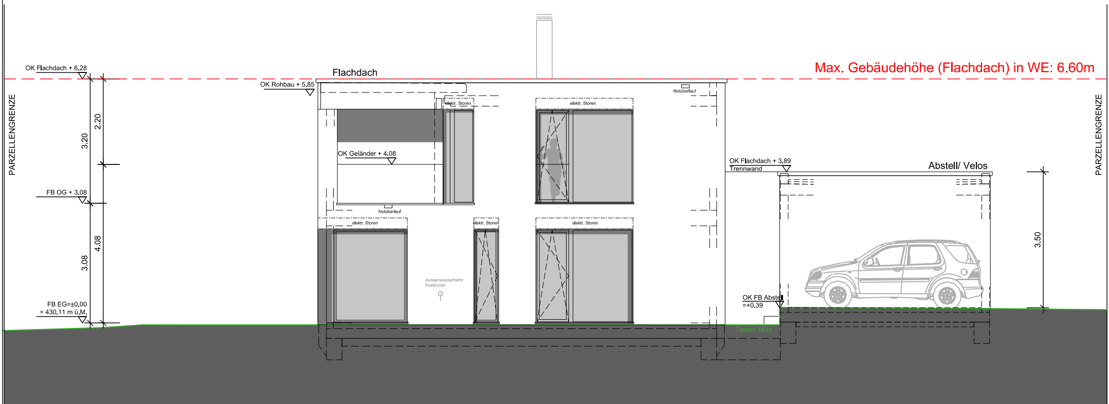
ANSICHT WEST
