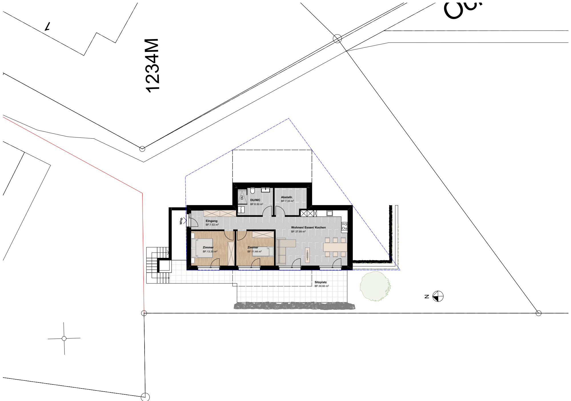
Grundriss Einliegerwohnung Untergeschoss, 1:200
