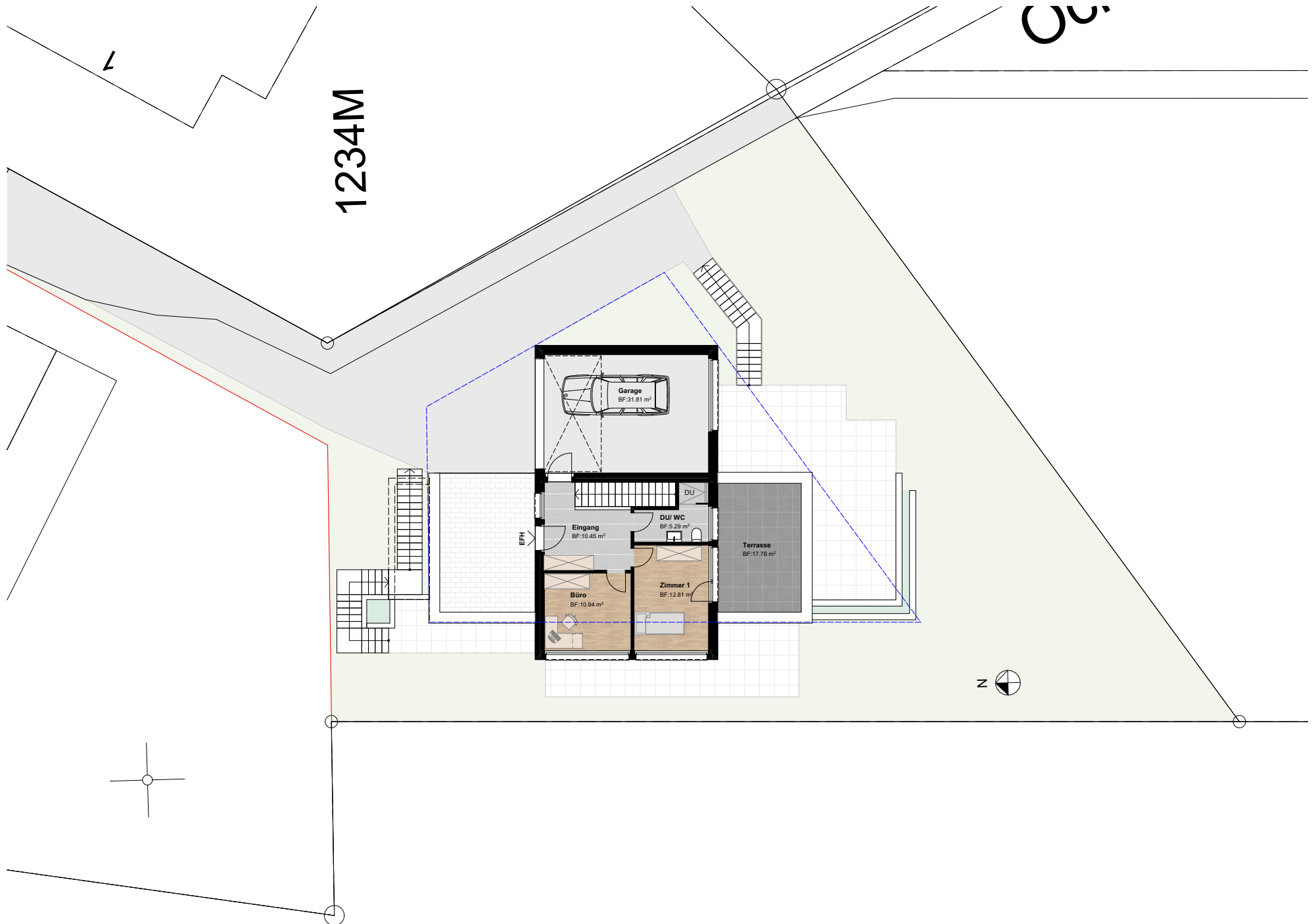
Grundriss EFH Obergeschoss mit Umgebung, 1:200
