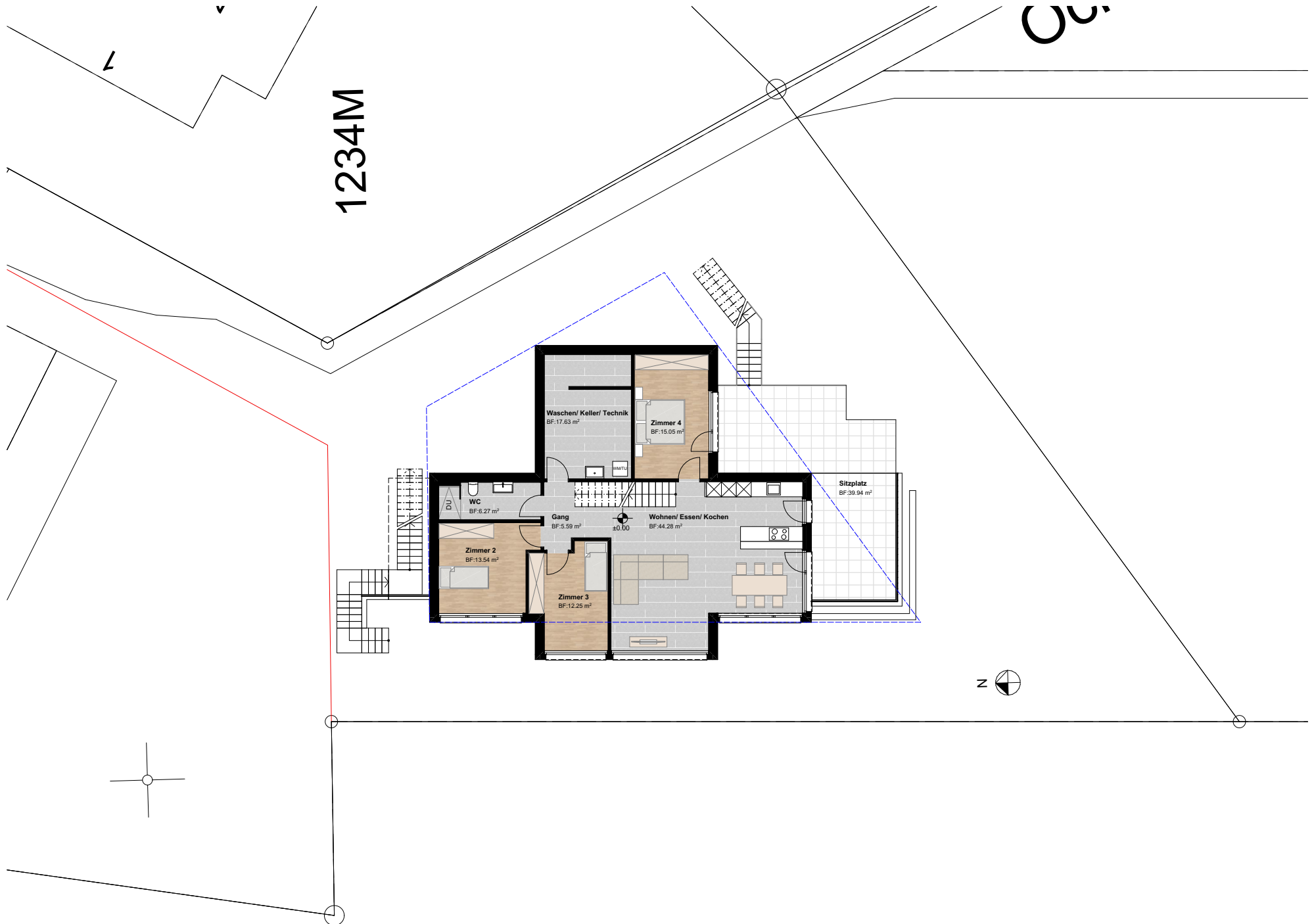
Grundriss EFH Erdgeschoss, 1:200
