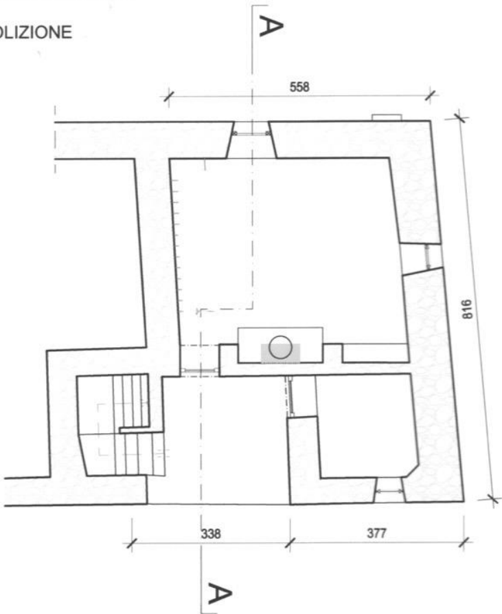
PIANTA PT
