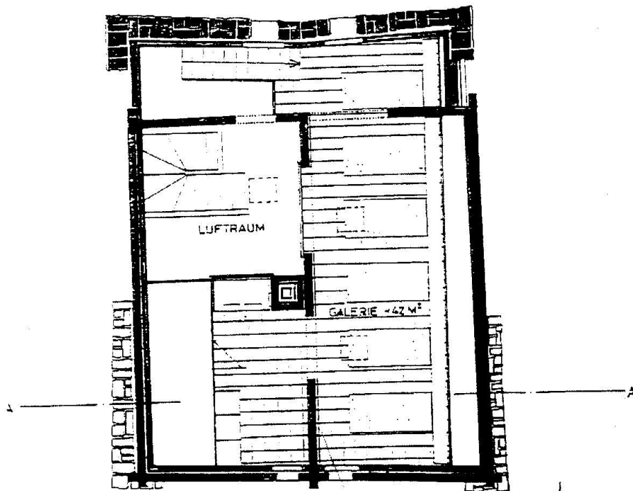
GRUNDRISS GALERIEGESCHOSS
