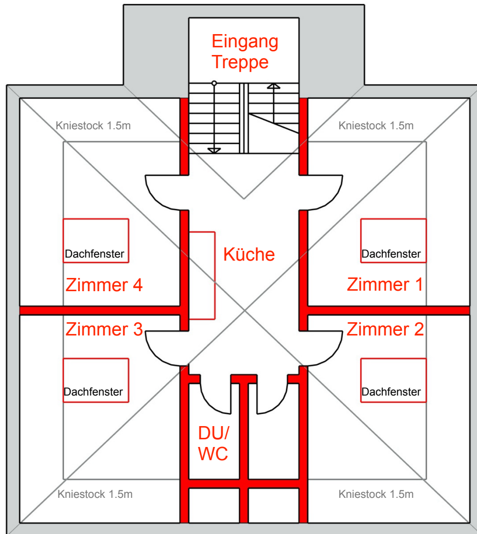
Dachgeschoss
