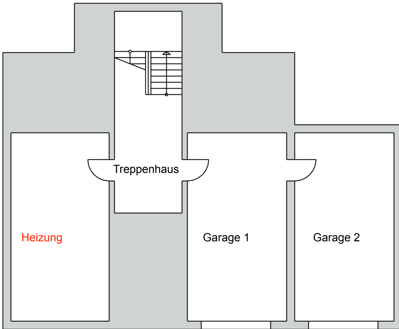
Untergeschoss
