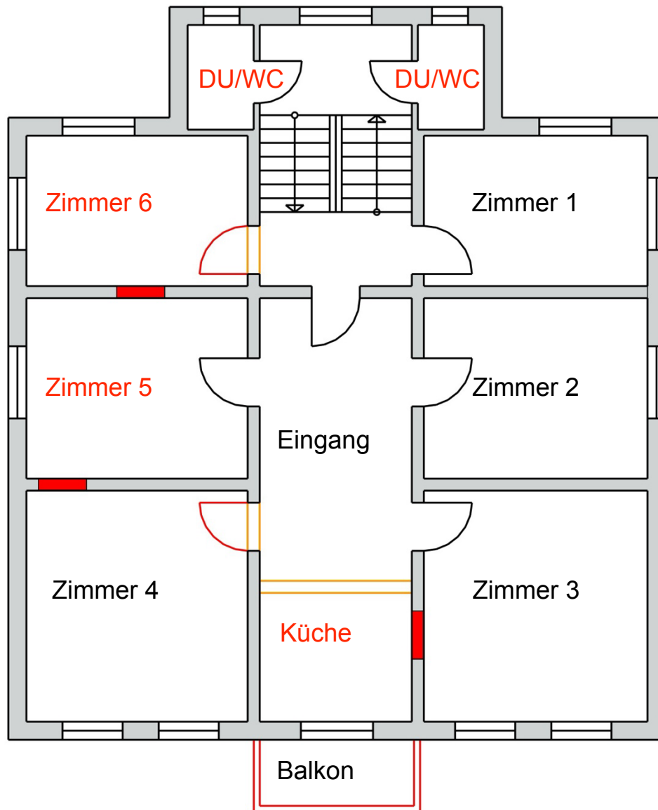
2. Obergeschoss
