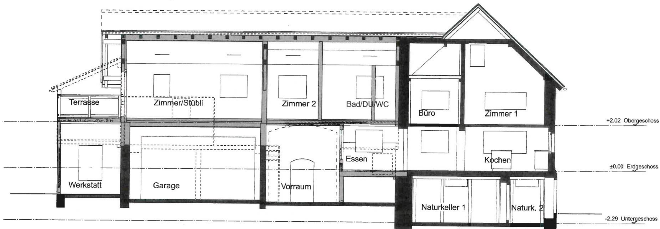
Schnitt A Mst.1:100
