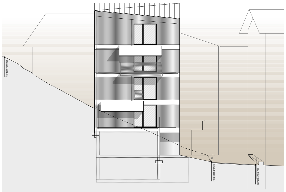
Ansicht Süden
