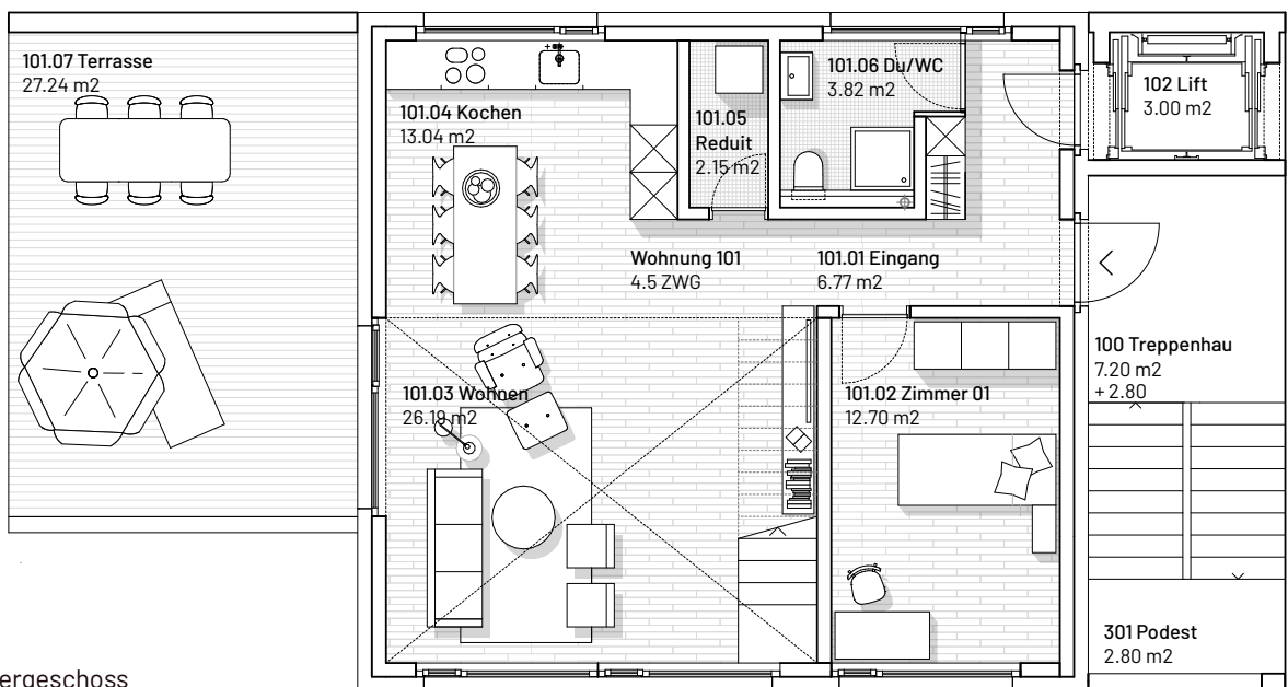
Grundriss 1. Obergeschoss
