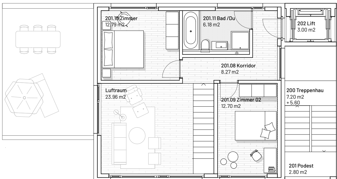
Grundriss 2. Obergeschoss
