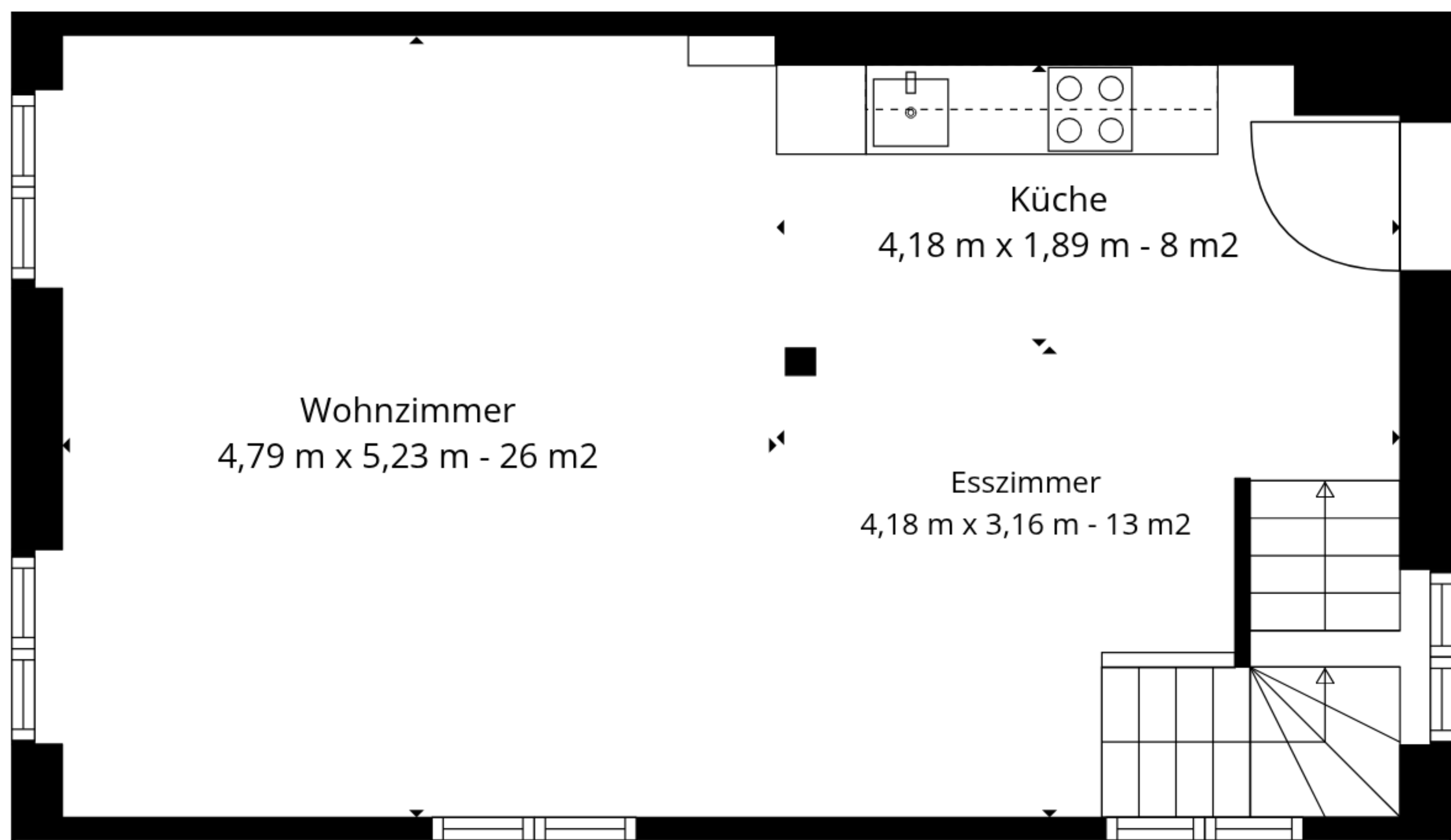
Erdgeschoss
