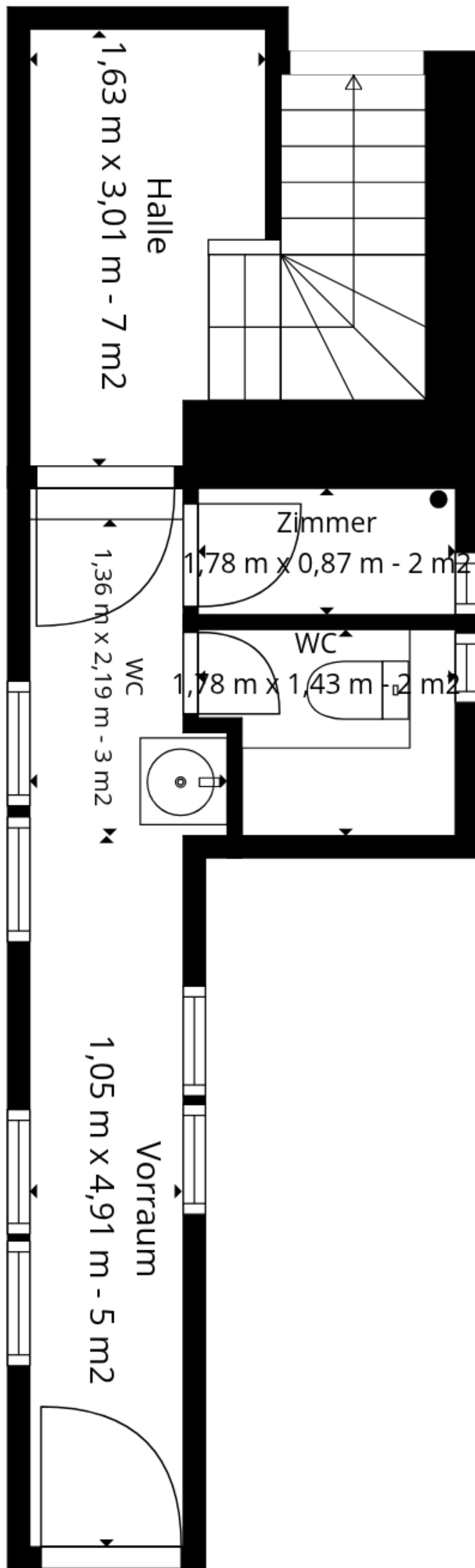
Keller
