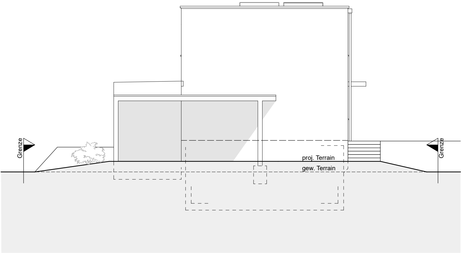
Ostfassade
