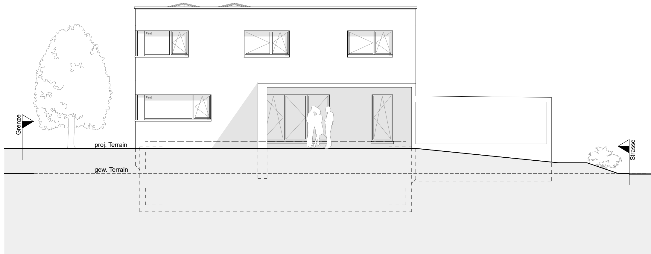
Südfassade
