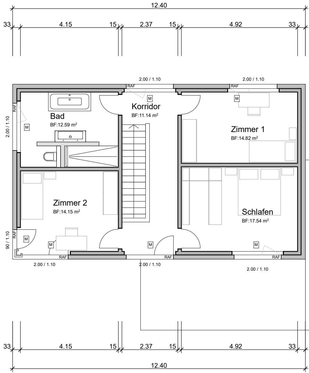
Obergeschoss
