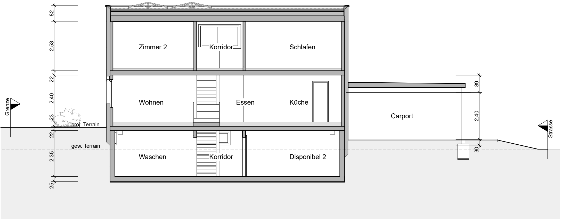
Schnitt
