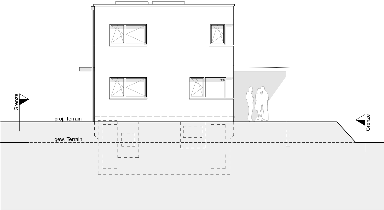
Westfassade
