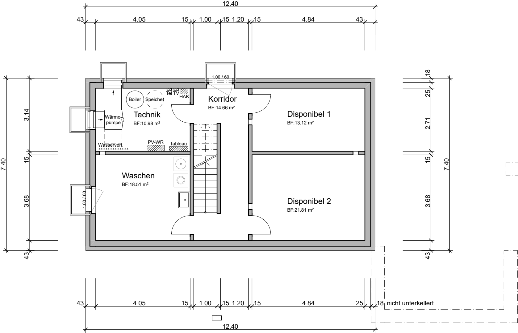
Untergeschoss
