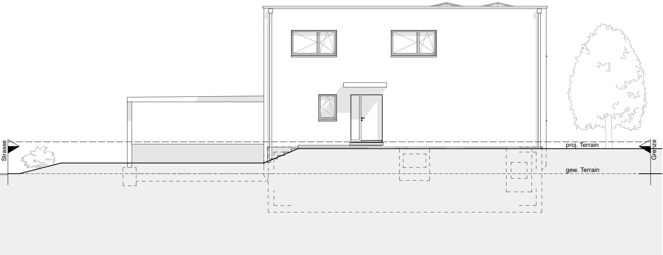
Nordfassade
