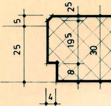
DETAIL KELLERFENSTER 1:10
