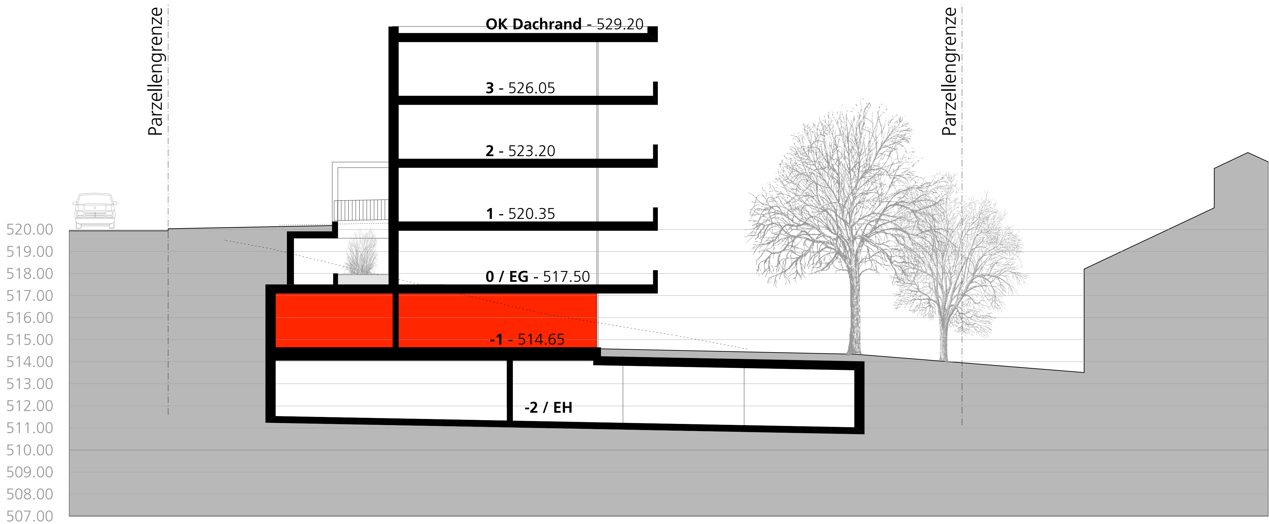
Schnitt B-B
