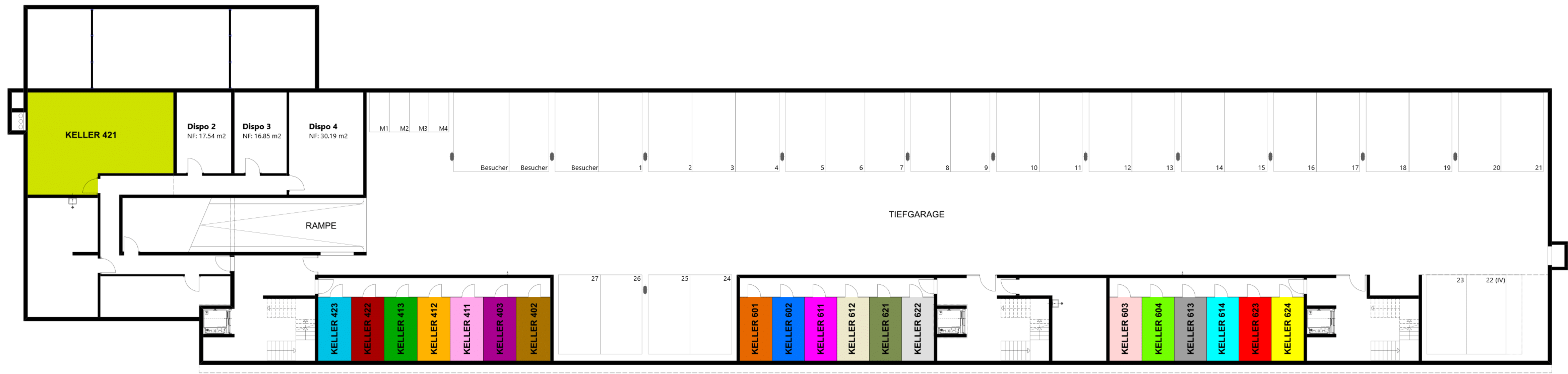
GRUNDRISS UG1
