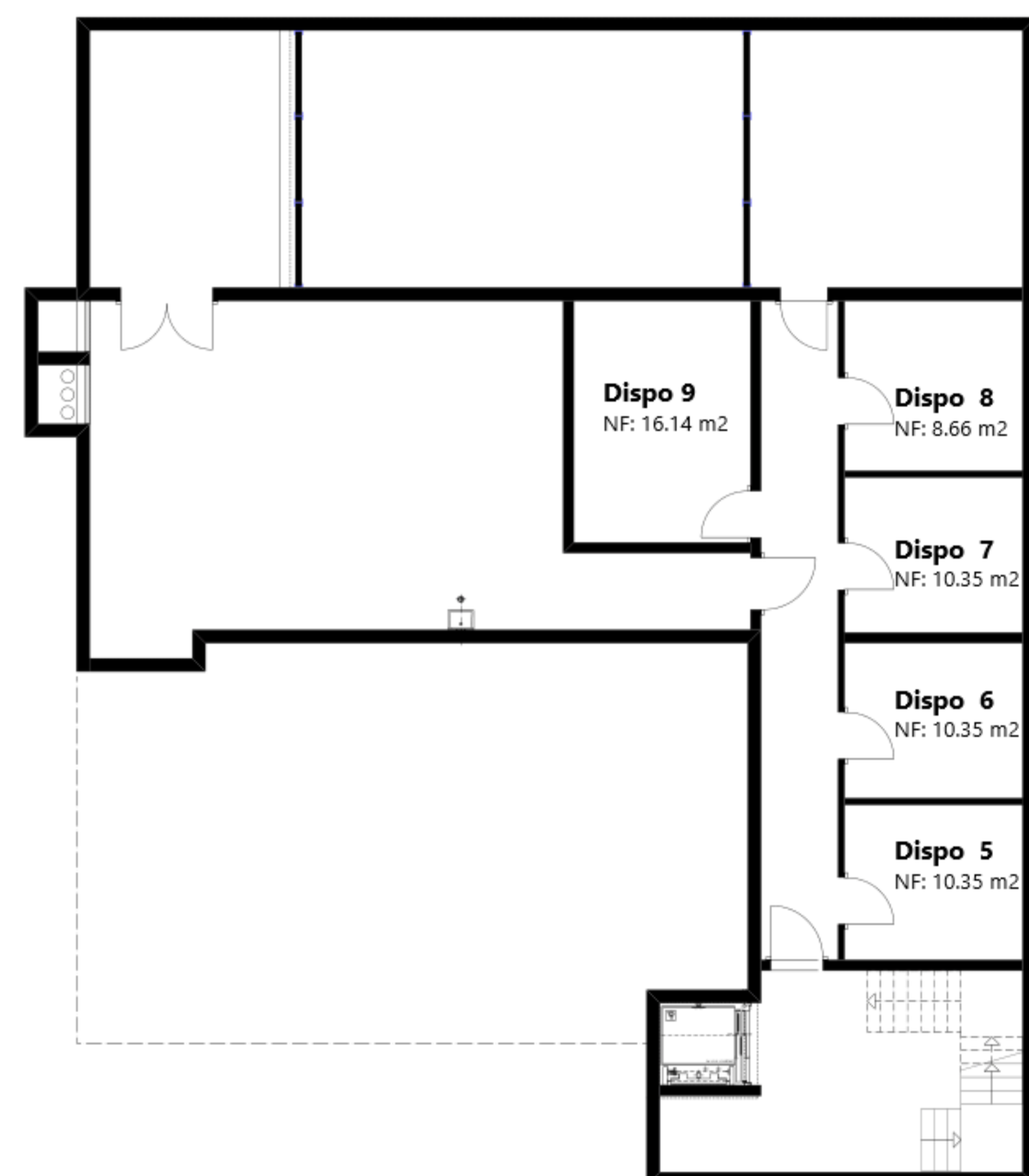
GRUNDRISS UG2
