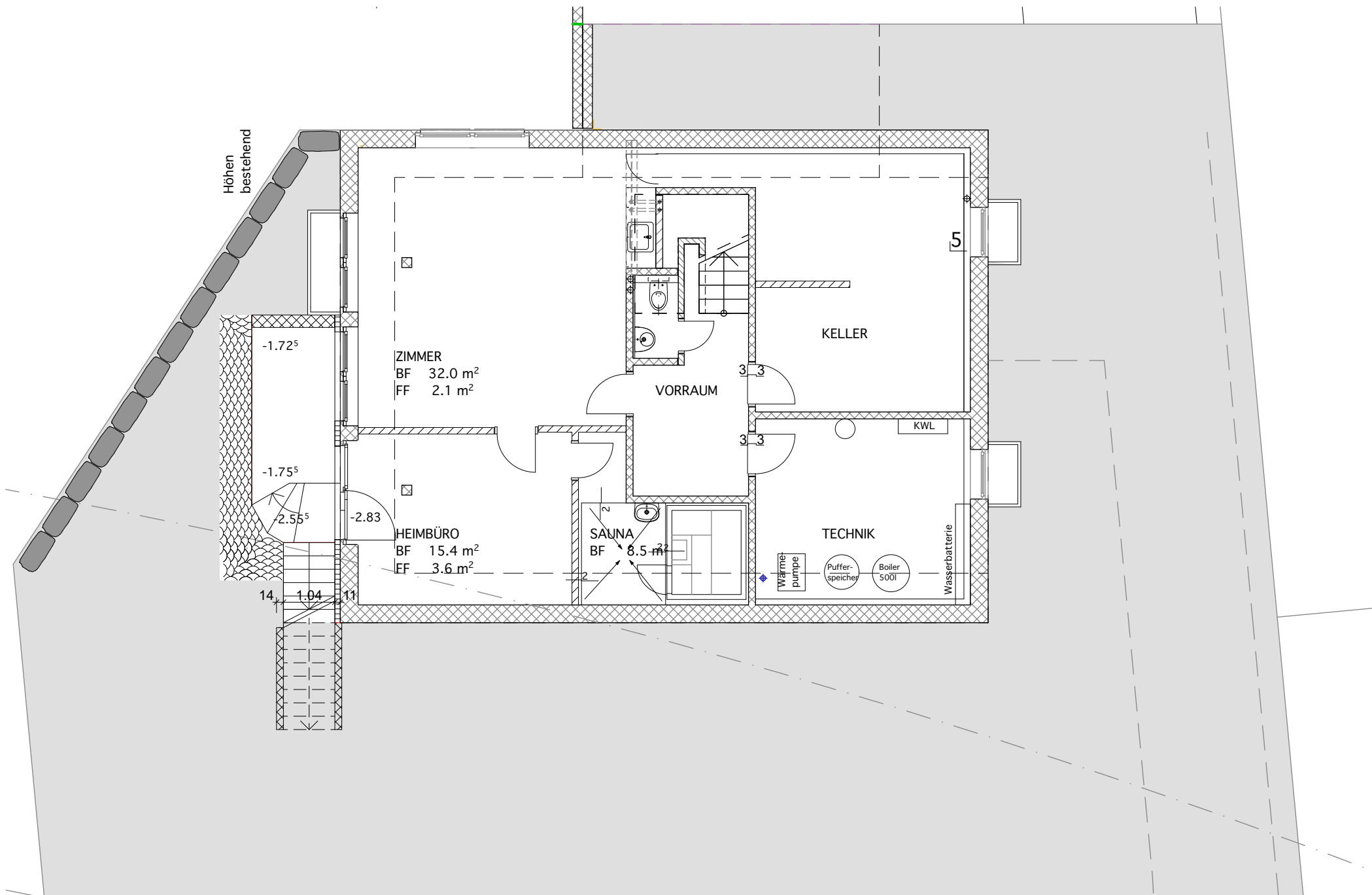
UNTERGESCHOSS – M. 1:100
