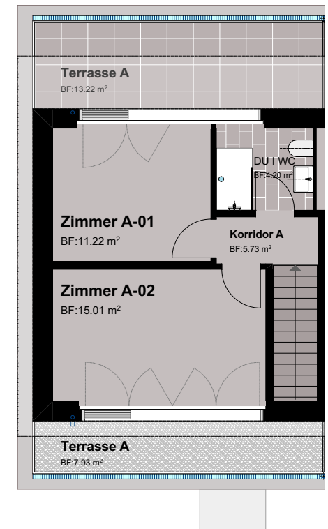
Obergeschoss
