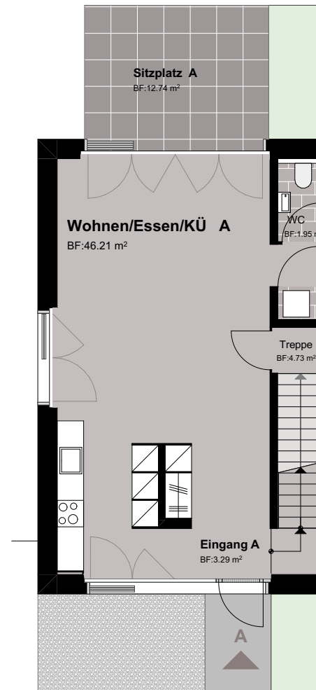
Erdgeschoss
