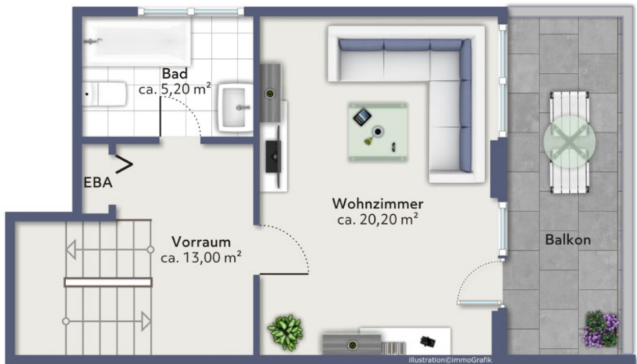
Grundriss 3. Geschoss
