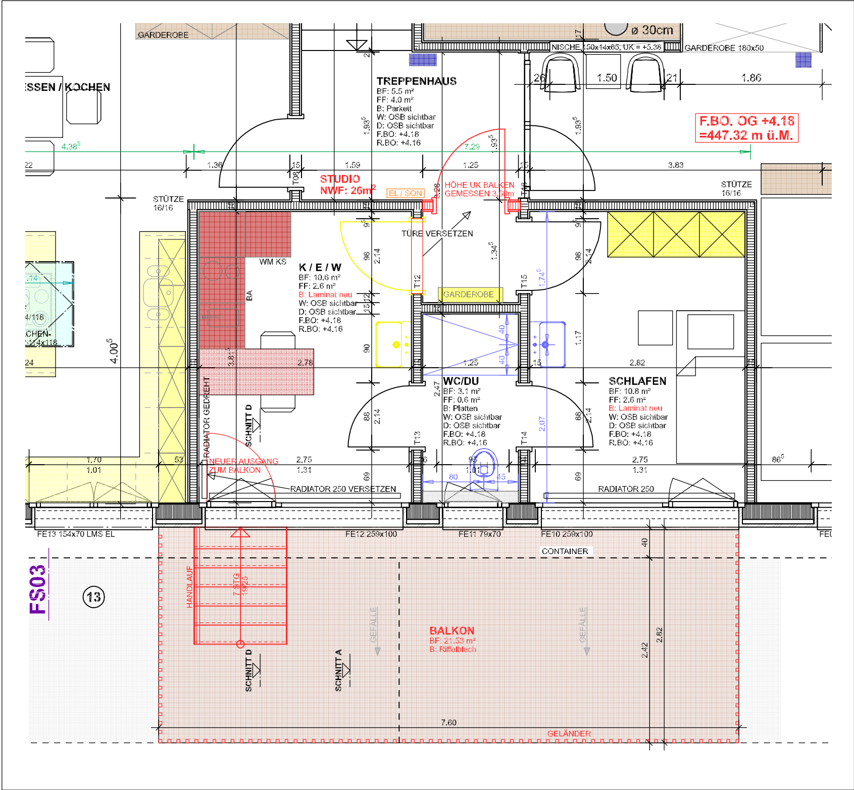
GRUNDRISS
