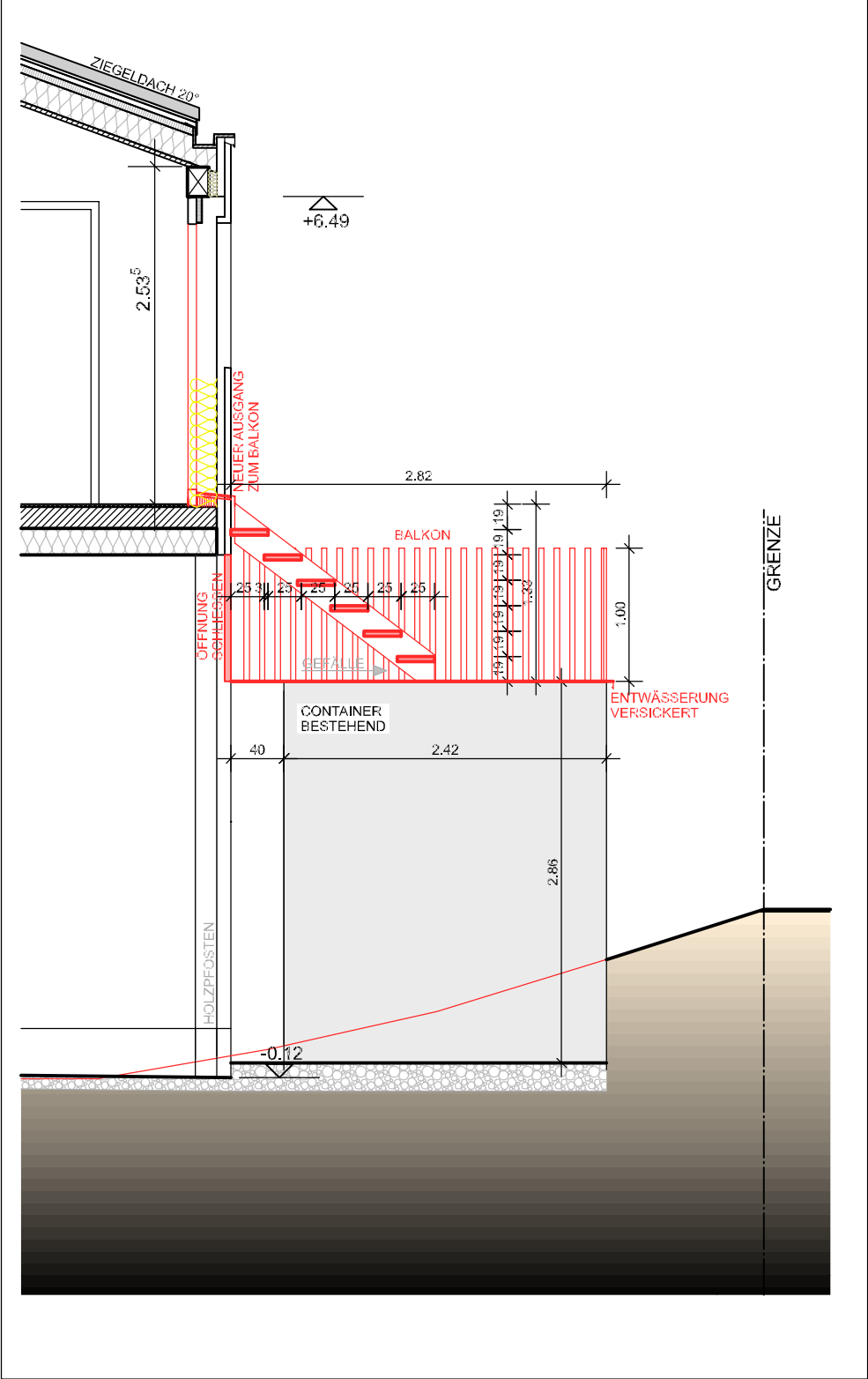
SCHNITT D
