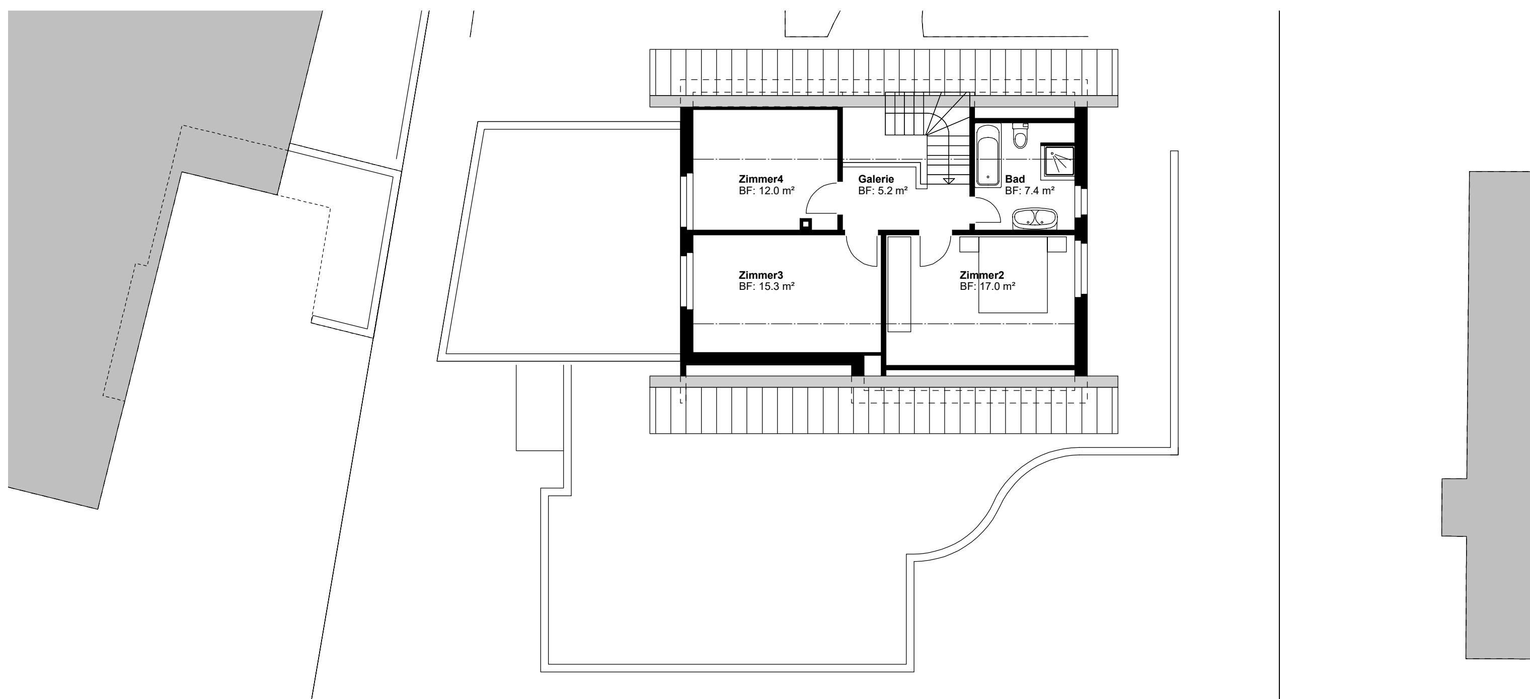
Dachgeschoss
