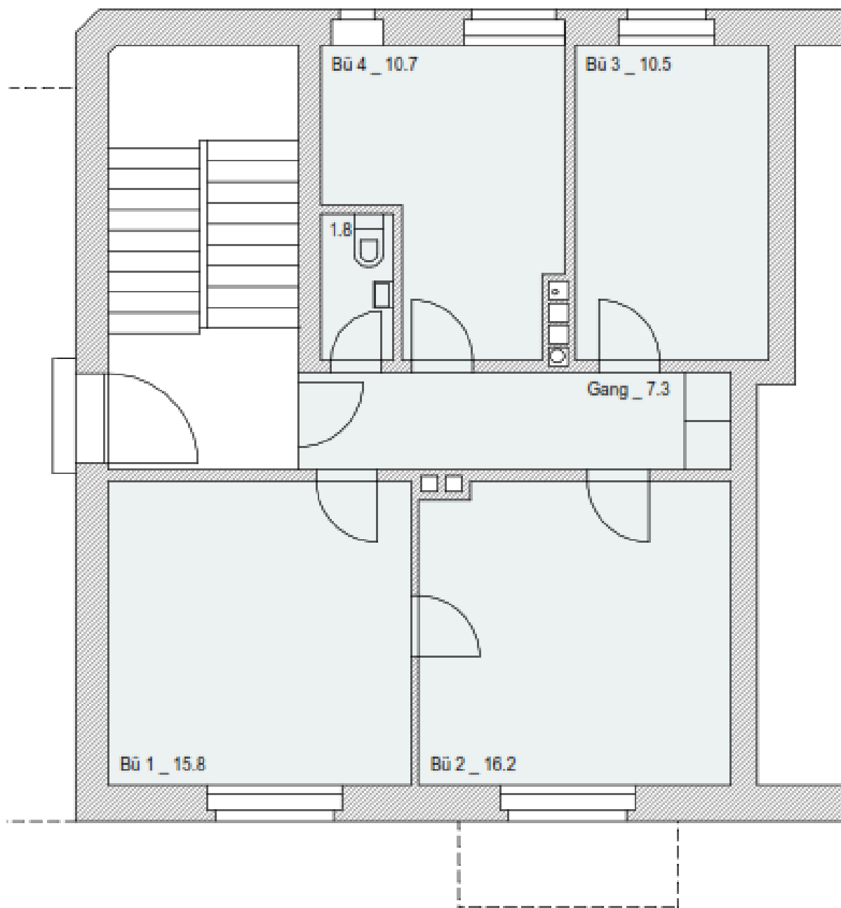
Erdgeschoss / Gewerbe / Büro
