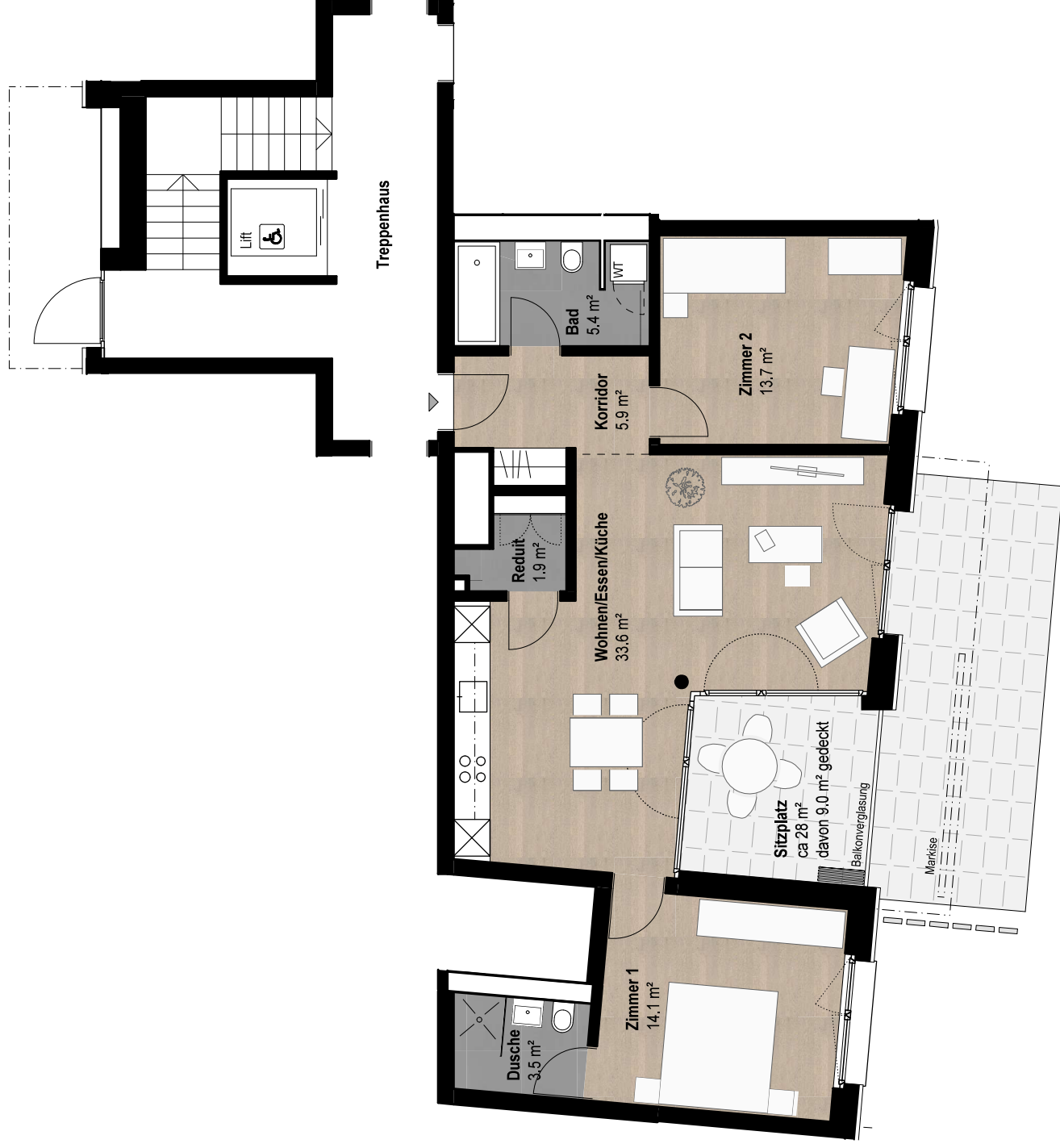
3.5-Zimmer-Wohnung R.003 Wohnfläche 78.0 m² Erdgeschoss
