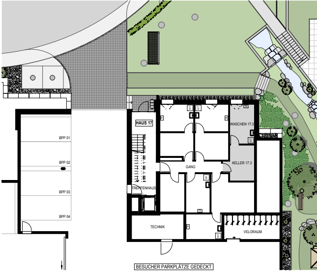
UNTERGESCHOSS 1:400
