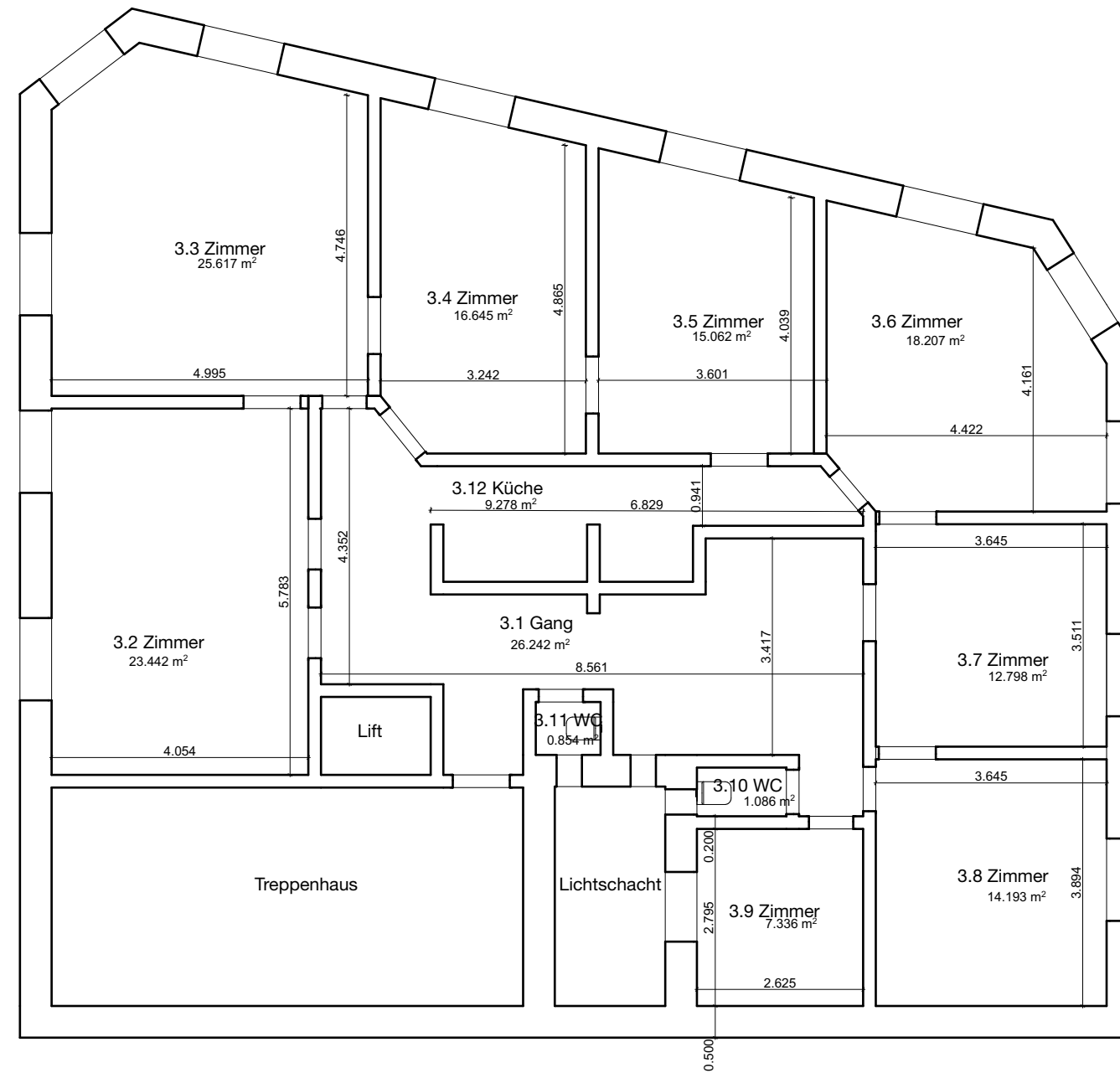
Grundriss 3. Obergeschoss 1:100
