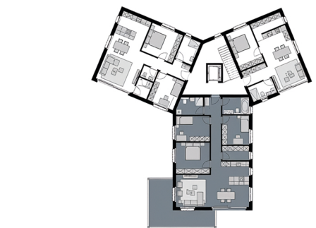
Geschossgrundriss
