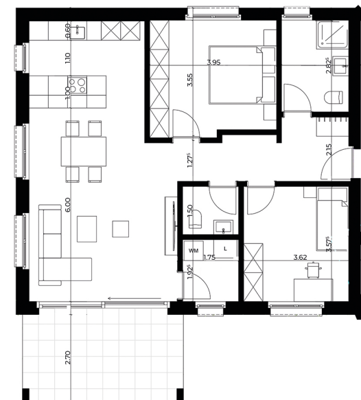
Wohnungsgrundriss
