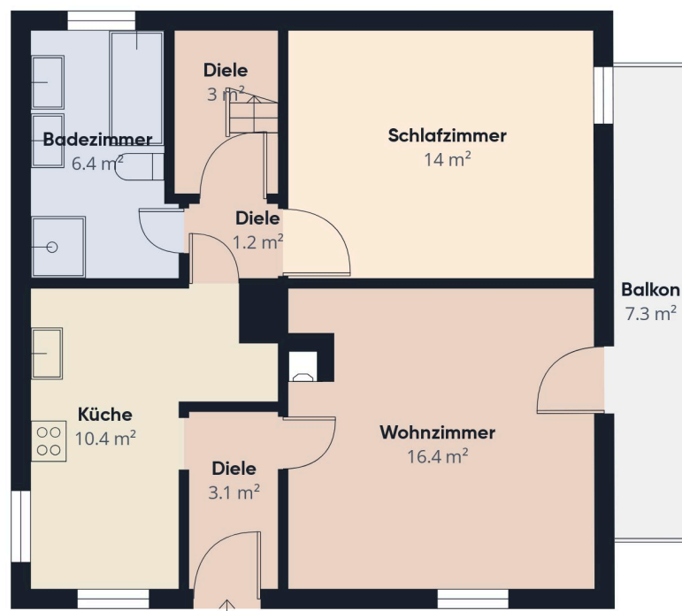
Etage 0
