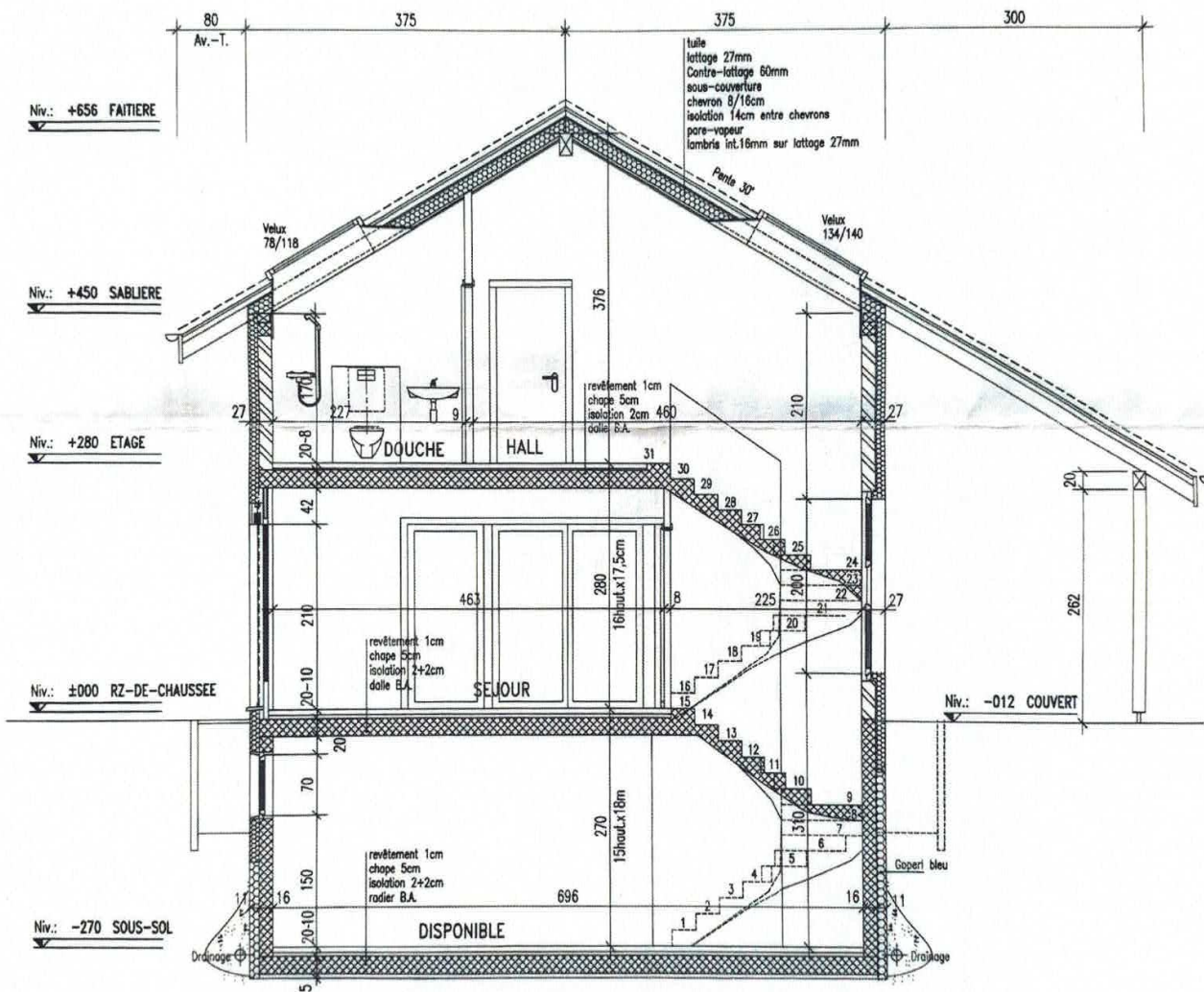
COUPE A-A
