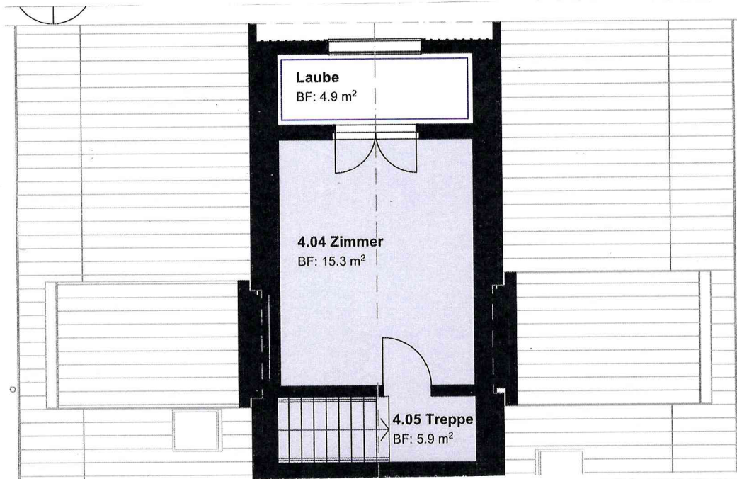
2. Dachgeschoss Mst: 1:100
