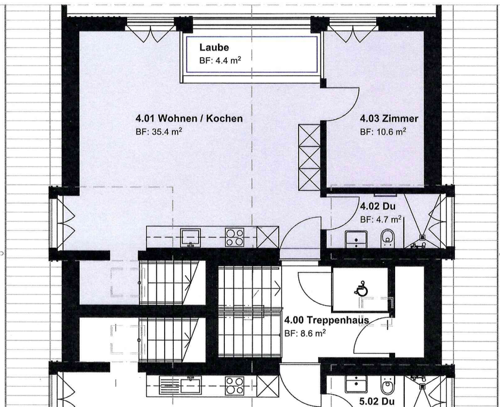
2. Dachgeschoss Mst: 1:100
