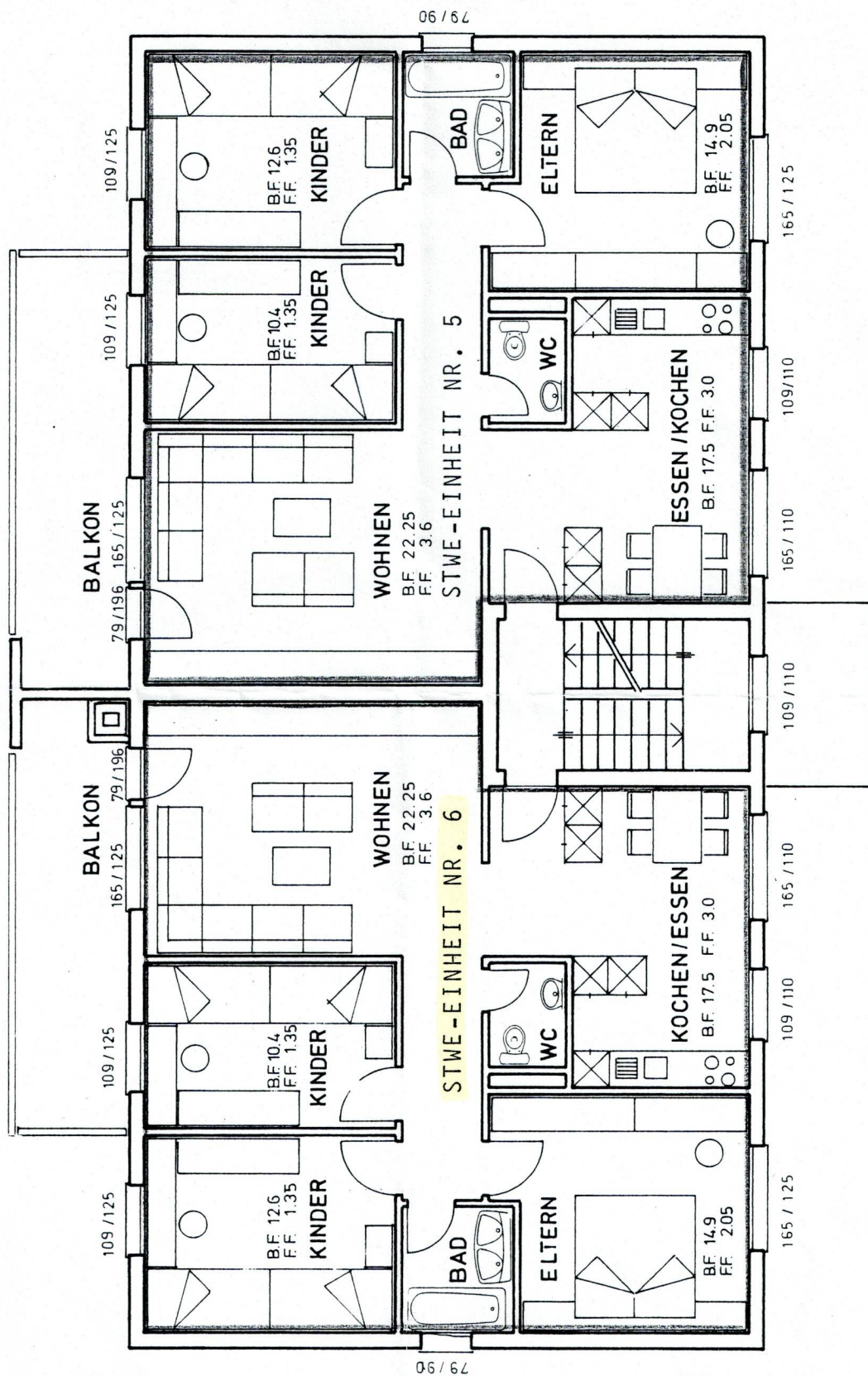
GRUNDRISS 2.OBERGESCHOSS
