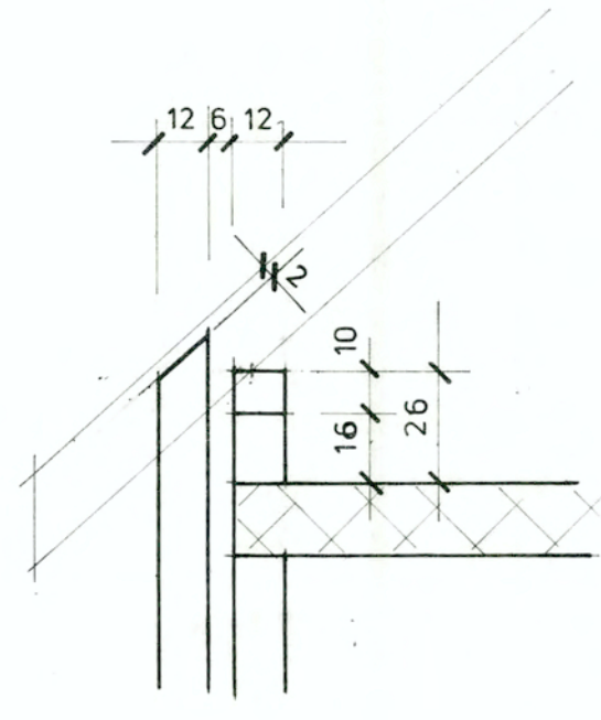
SCHNITT D-D
