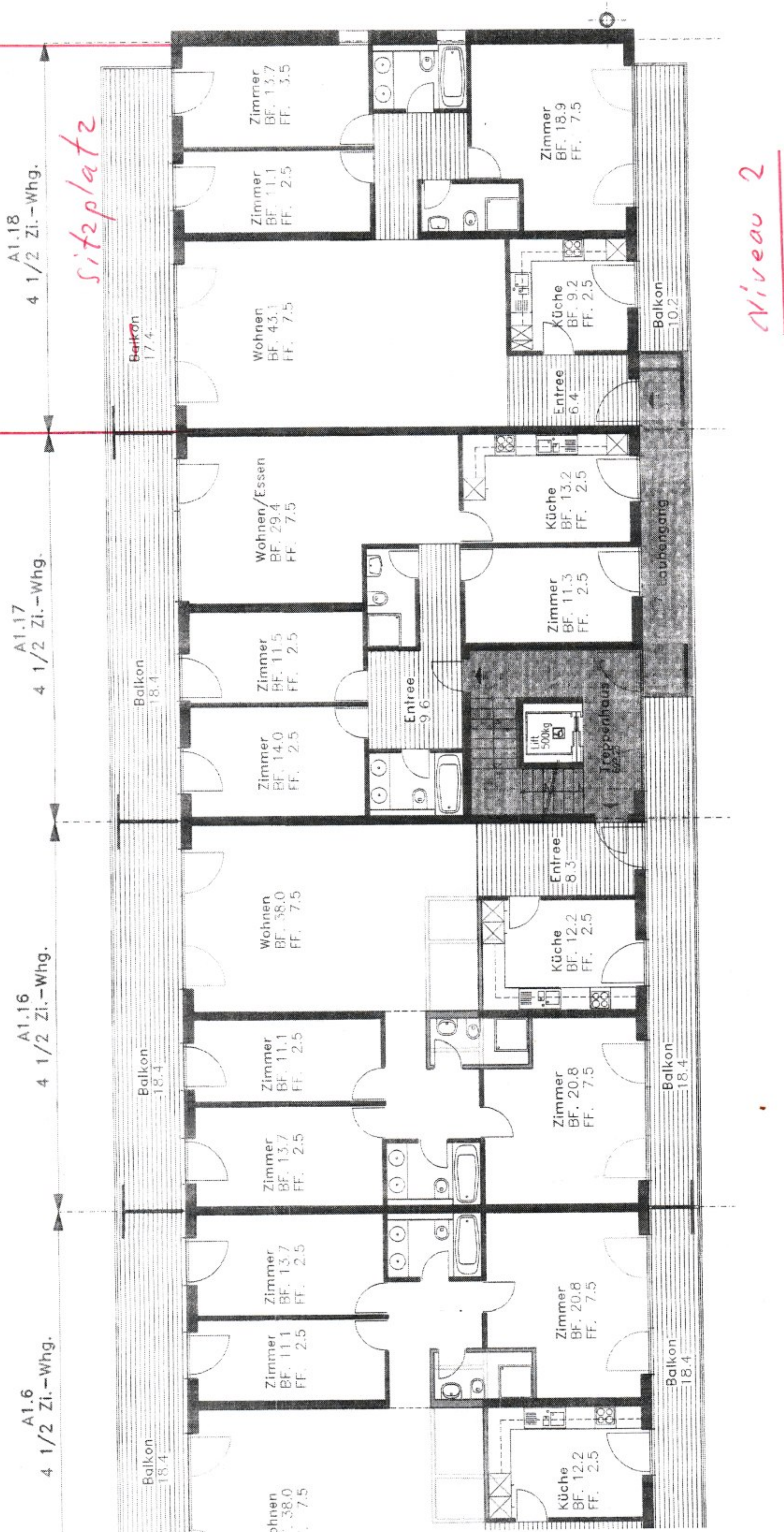
Haus A1 Niveau (3) 1:100
