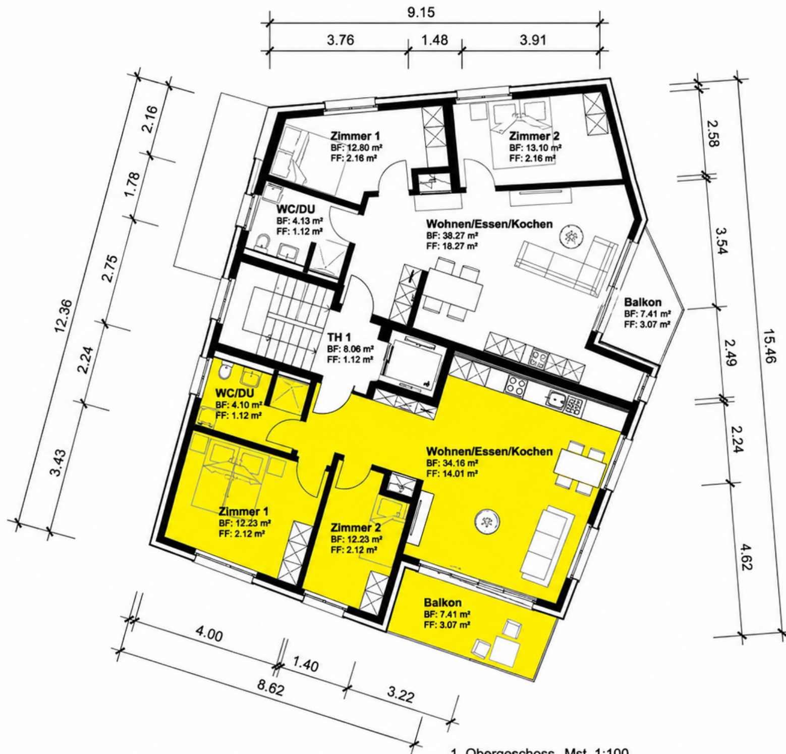
1. Obergeschoss Mst. 1:100
