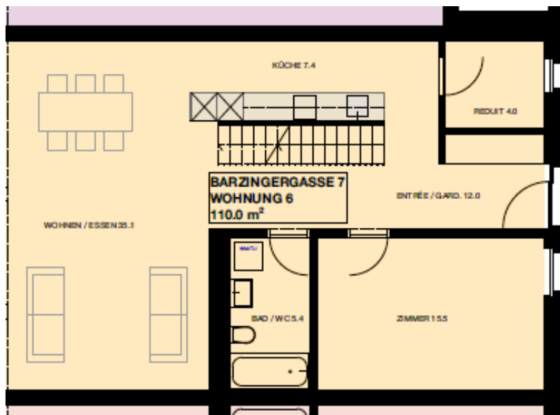
2. OG
