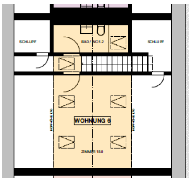
Dachstock
