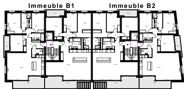
Plan repérage
