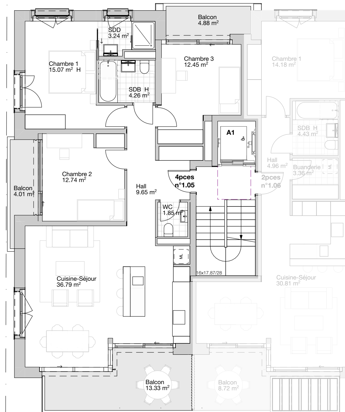
4 Pièces n°1.05
